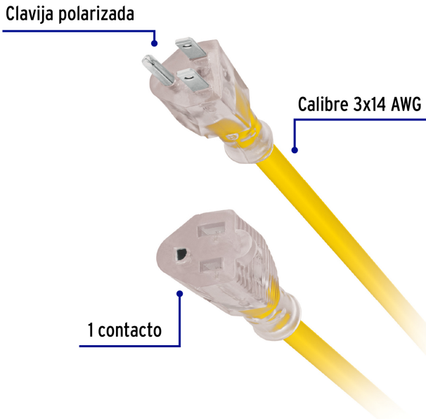
EMPAQUE INDIVIDUAL
